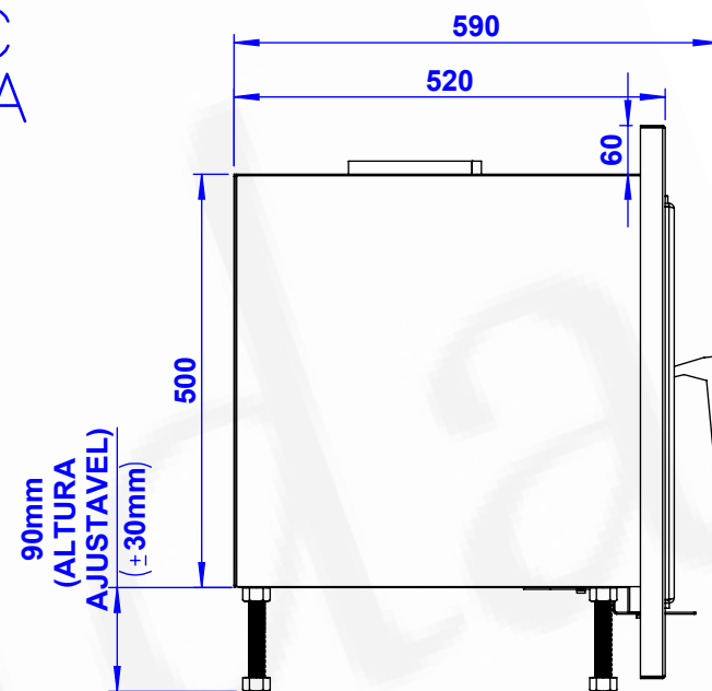
VISTA LATERAL
