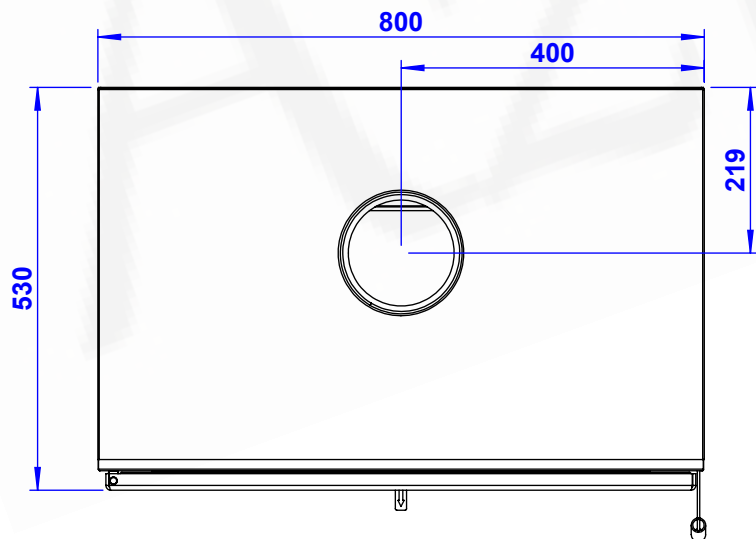
VISTA SUPERIOR
